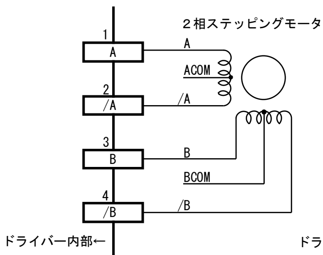
接続例 a) フルコイル接続
