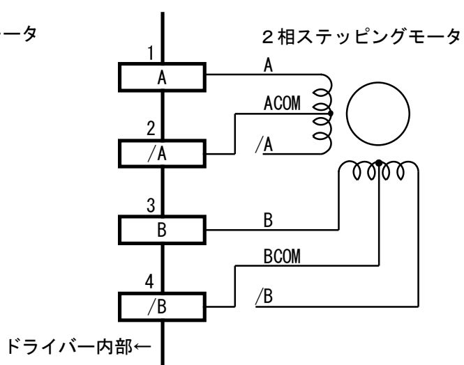
接続例 b) ハーフコイル接続
