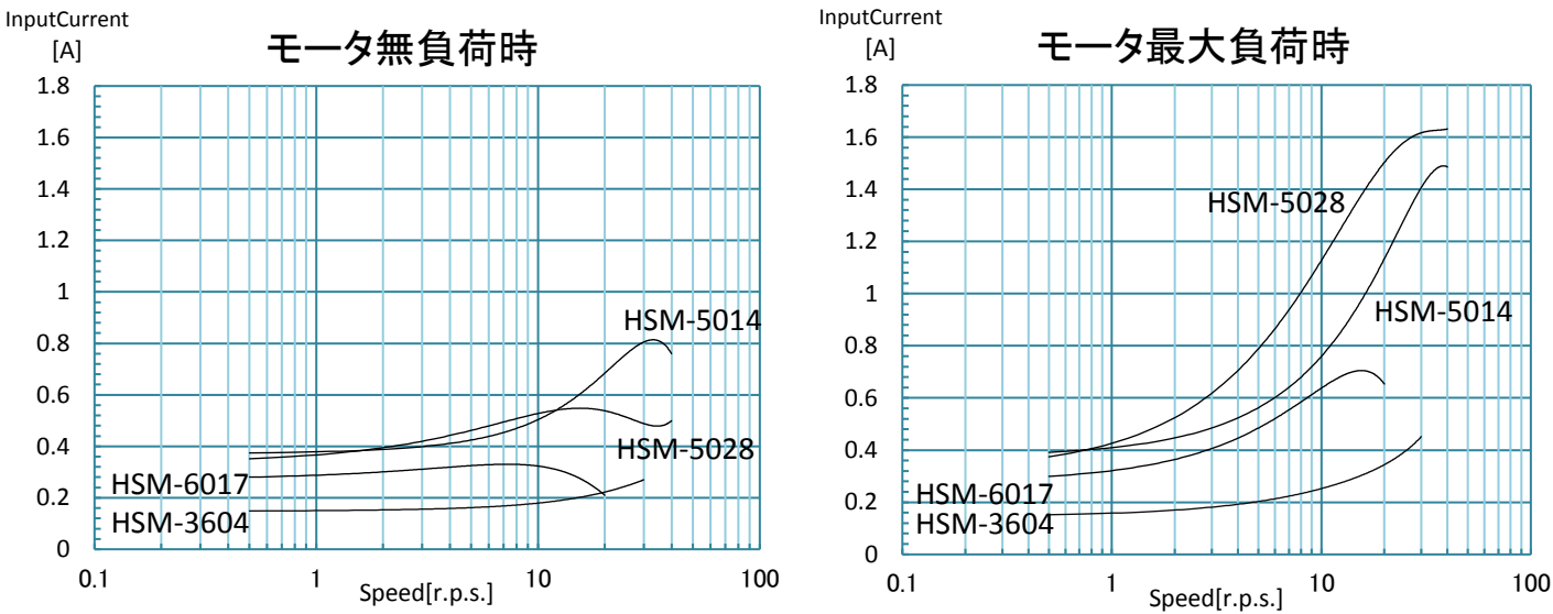
入力電流・速度曲線 (弊社ドライバ AK-BX2120-2. 5P、DC24V、分割数 10, 000P/R)
