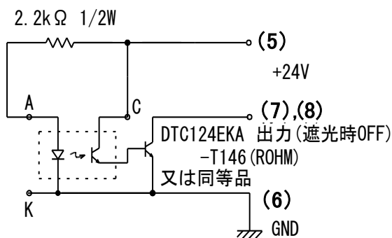
(フォトマイクロセンサ；OMRON EE-SX1103 又は同等品)
