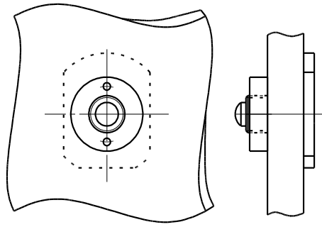
付属するナットの締め付けトルクは 1.0 N・m 以下として下さい。
